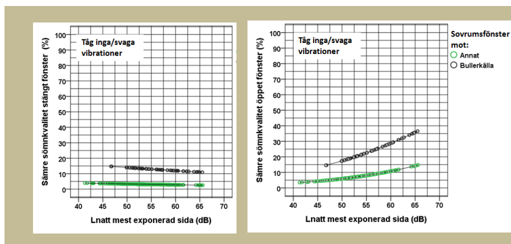
Figur 6.6. Områden med inga/svaga vibrationer. Predicerat värde för andel med försämrad sömnkvalitet p.g.a. tågbuller i relation till ljudnivå i L_{natt} för personer med sovrumsfönster mot järnvägen (svart kurva) respektive mot annat håll (grön kurva). Vänster figur visar sömnstörning vid stängt fönster och figuren till höger visar sömnstörning vid öppet fönster.
