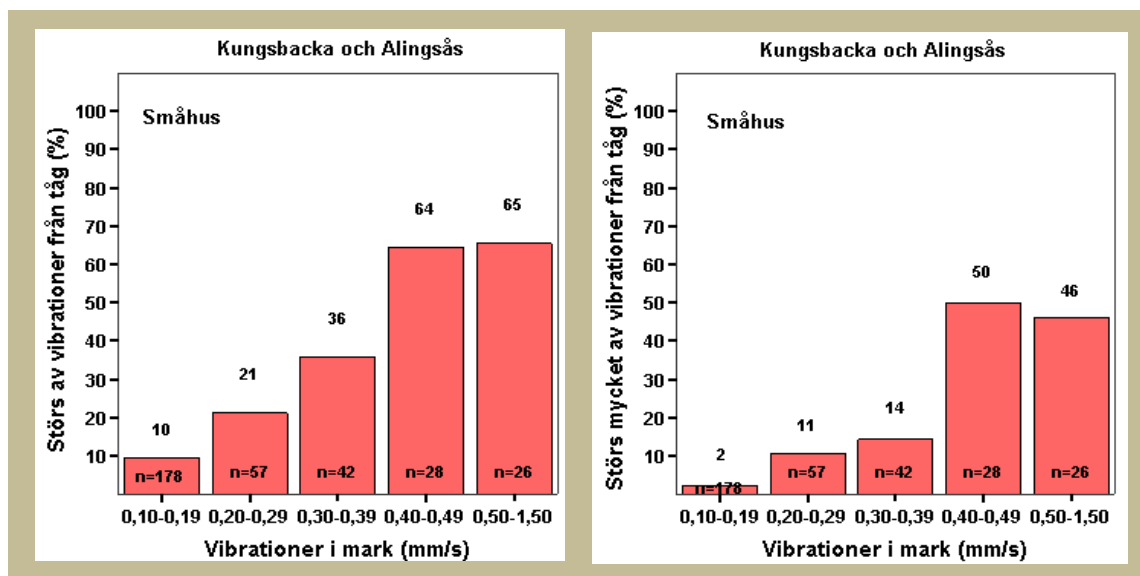
Figur 5.3. Andel (%) av boende i småhus som är störda (vänster figur) respektive mycket störda (höger figur) av tåg vibrationer i relation till vibrationsnivå i mark i Kungälv och Alingsås (n=331).
