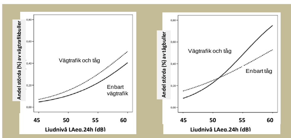
Figur 7.3. Vänster: Samband mellan störning av vägtrafikbuller och ljudnivå ( L_{Aeq,24h} ) för personer med lika exponering för vägtrafik och tåg (streckad kurva) och för personer exponerade enbart för vägtrafik (heldragen kurva). Höger: Samband mellan störning av tågbuller och ljudnivå ( L_{Aeq,24h} ) för personer med lika exponering för tåg- och vägtrafikbuller (heldragen kurva) och för personer exponerade enbart för tågbuller (streckad kurva).
