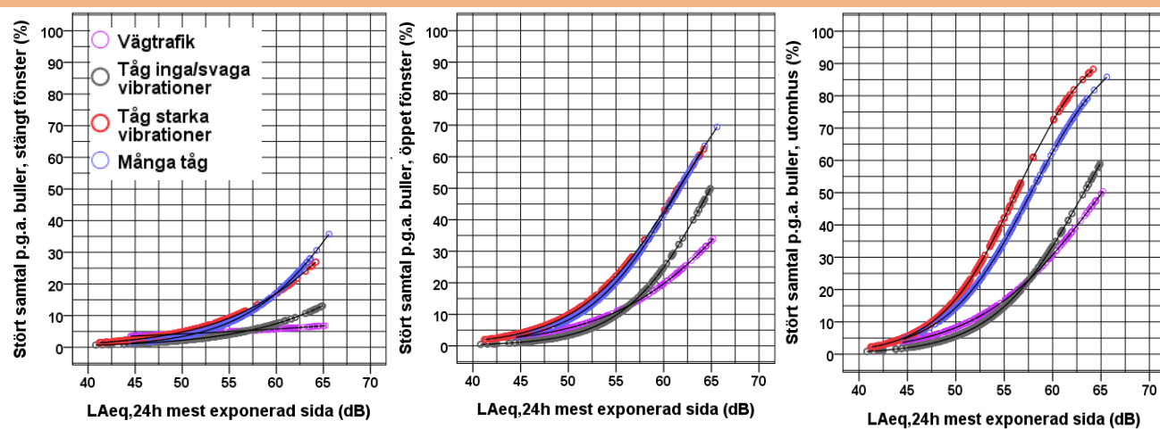
Figur 4.6. Samband mellan störning av samtal (andel i % >3) och ljudnivå i L_{Aeq,24h} för olika undersökningsområden vid stängt fönster (vänster), öppet fönster (mitten) och utomhus vid uteplats (höger).
