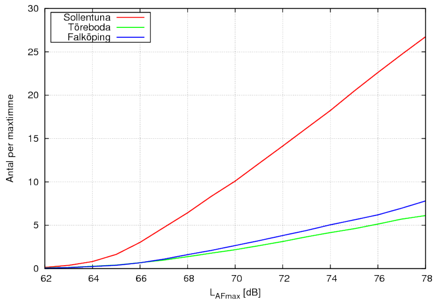
Figur 3.5. Beräknat antal passager som överstiger 70 dB vid maxtimme som funktion av beräknad L_{AFmax} .
